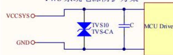
TWS 系统电源防护方案
