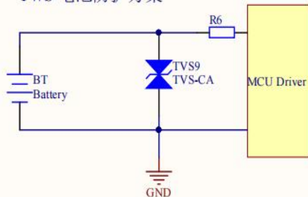
TWS 电池防护方案
